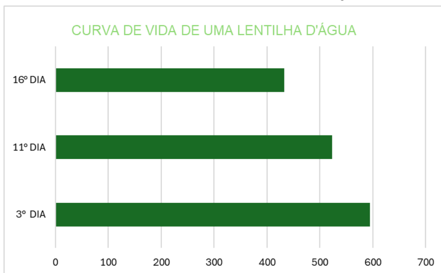
Gráfico 1 – Curva de vida de lentilhas D'água.
