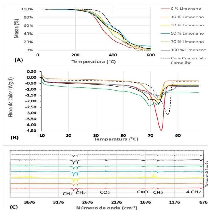
Figura 1. Análises térmicas - (A) TGA, (B) DSC - e dos grupos funcionais - (C) FTIR - da cera purificada.
