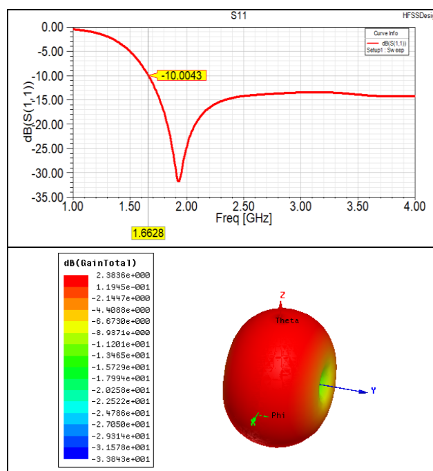
Figura 3. Análise da perda de retorno e Padrão de radiação para 1.6628 GHz na antena monopolo circular.
