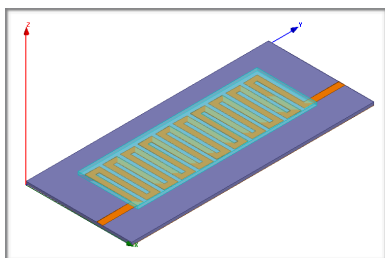
Figura 1. Estrutura zig-zag junto com a camada de polímero
