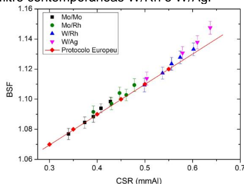
Figura 1. Resultados de simulação para o BSF.
