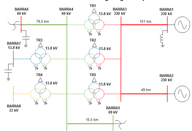
Figura 1. Sistema Elétrico Real em Estudo para Aplicação da Proteção Diferencial de Barras.
