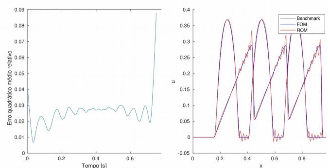
Figura 1. Erro quadrático médio relativo do modelo de ordem completa e do modelo de ordem reduzida (à esquerda) e comparação do padrão com modelo de ordem completa e do modelo de ordem reduzida com m = 21 modos espaciais (à direita).
