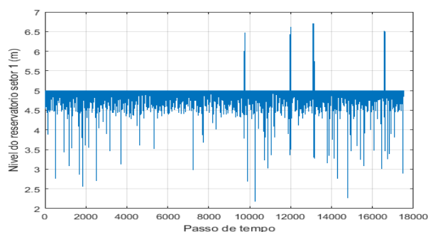
Figura 1. Série temporal de nível de reservatório com anomalias programadas
